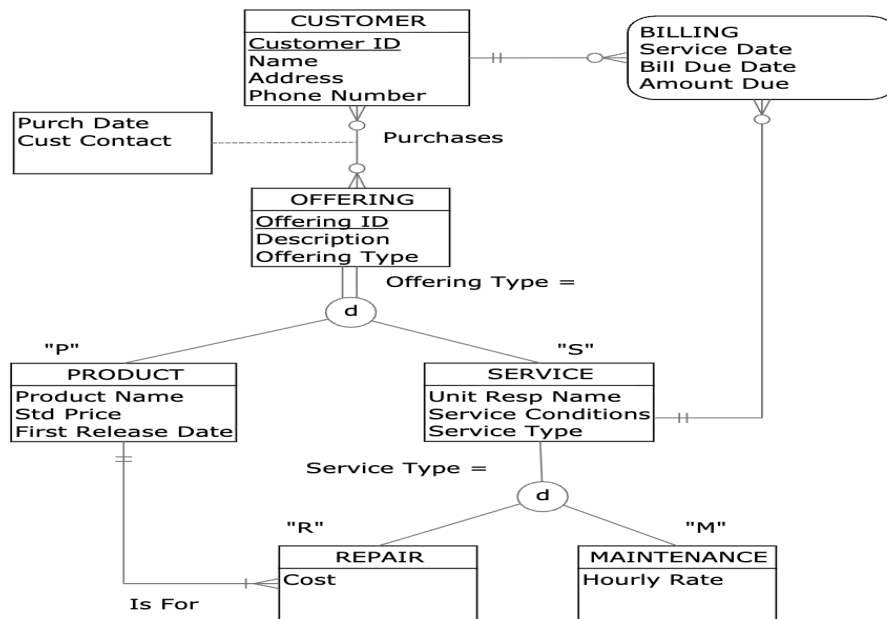
EER Diagram 1
